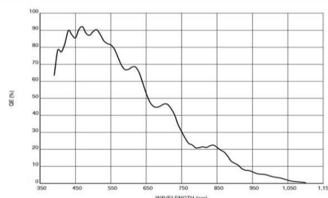
MV-CU050-30GM 响应曲线
