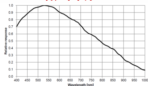
MV-CU060-10GM 响应曲线
