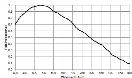
MV-CU060-10UM 量子效率
