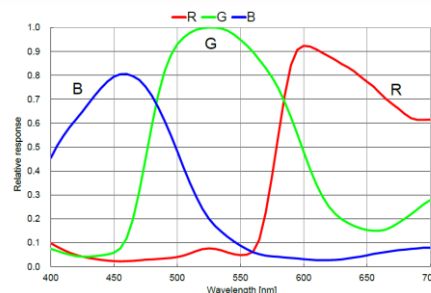
MV-CU060-10UC 量子效率
